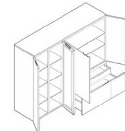
Vitrina de 150 x 137 con zócalo ACABADO CHAPA DE ROBLE NATURAL BLANQUEADO / METALIC.
